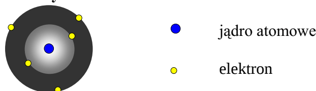
uproszczony model atomu
