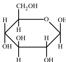
\beta -D-glukopiranoza
