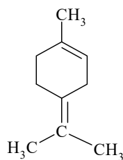
IV terpinolen
